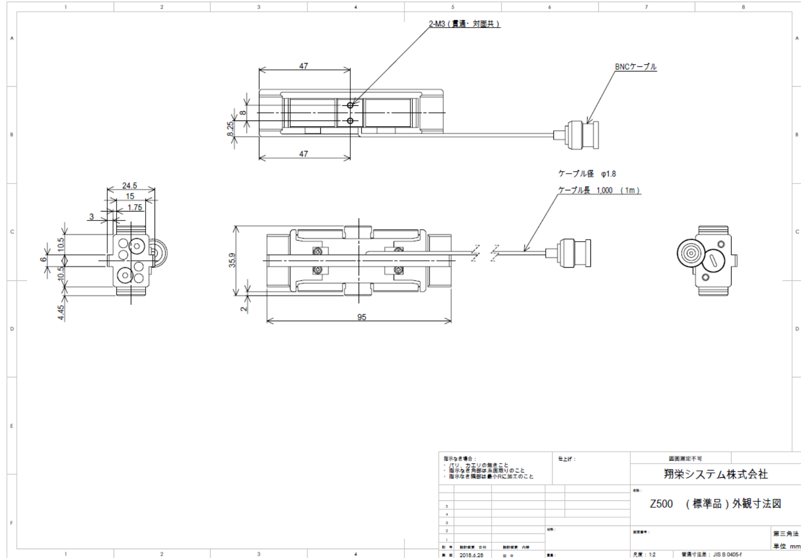
外観寸法図
