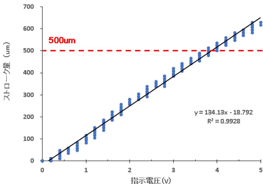
図2 Z500 の最大ストローク(変位量)と制御電圧の関係 (-30V~150V 印加時)
