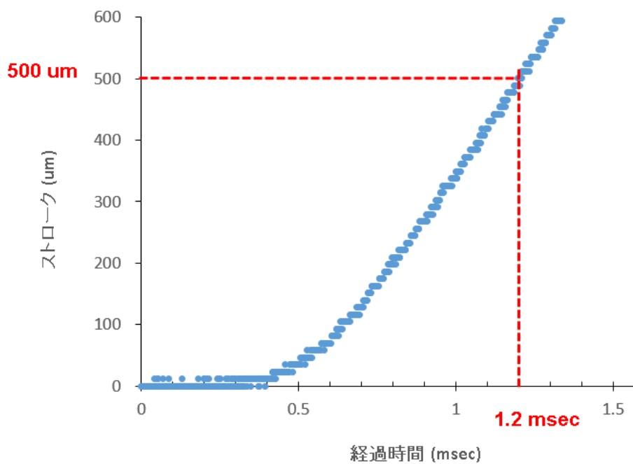
図3 Z500 の到達時間とストロークの関係
