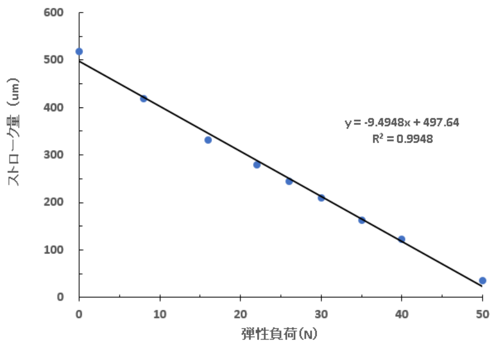
図 4 Z500 の弾性負荷とストロークの関係
